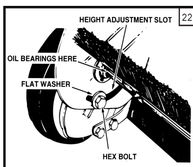
Abb. 22: Höhenverstellung
