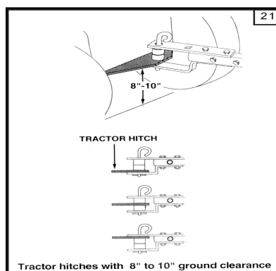
Abbildung 21: (Traktor Höhe 20-25 cm über dem Boden)
