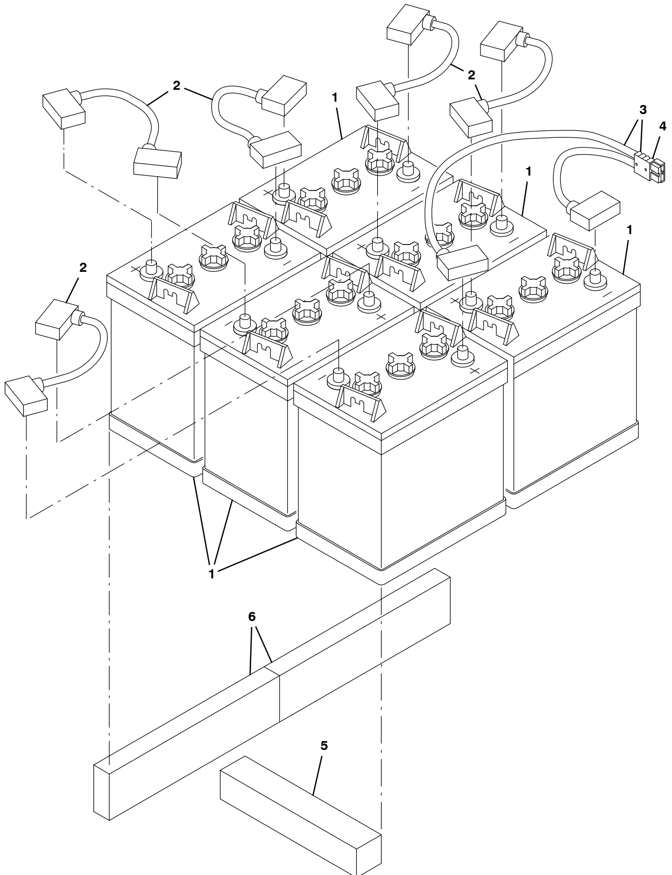
Fig. 17 – Battery Group, 185AH — Batterie Gruppe, 185AH — Groupe Batteries, 185AH
