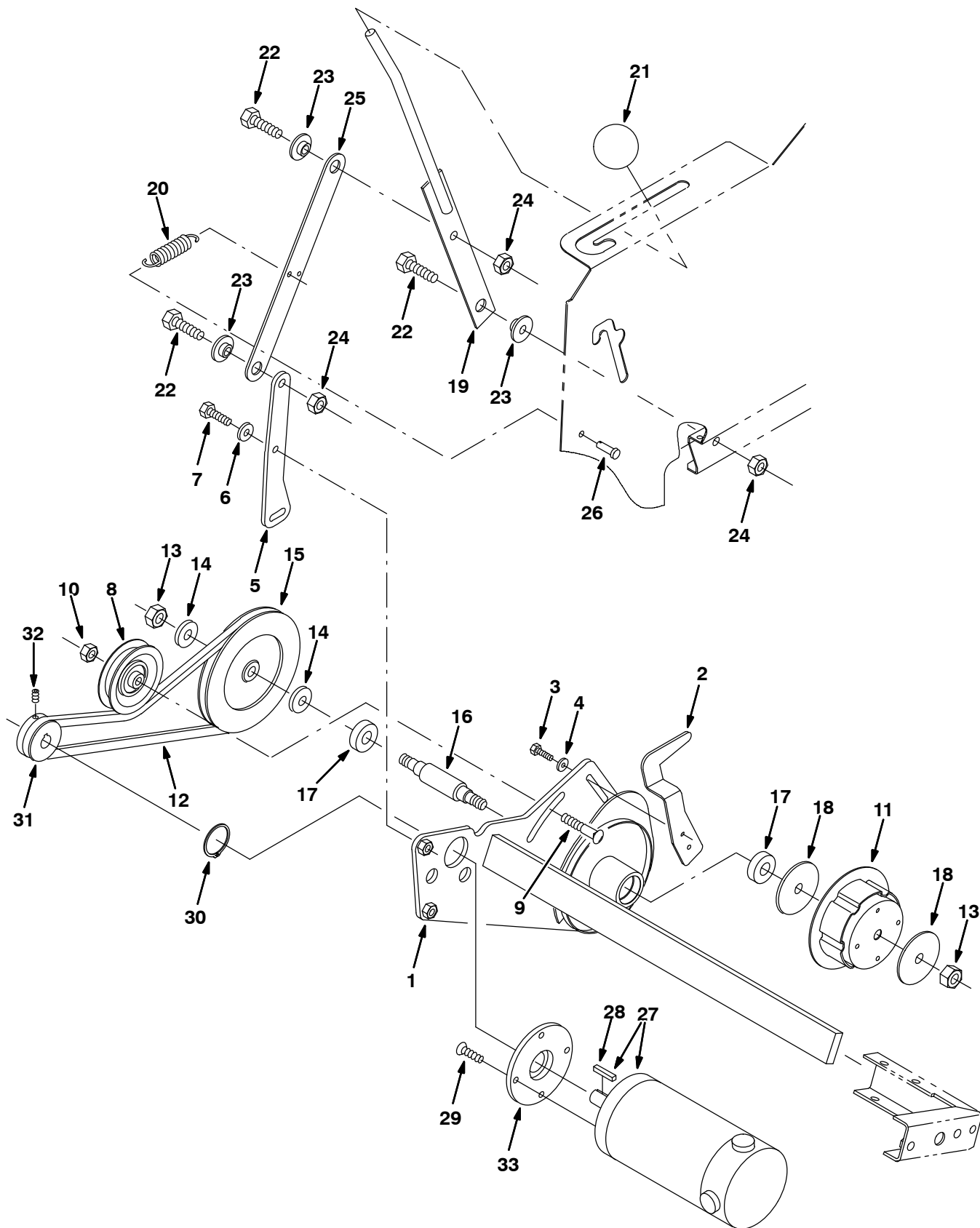
Fig. 21 – Main Brush Drive Group — Kehrwalzeantrieb-Gruppe — Groupe entraînement de la brosse principale
