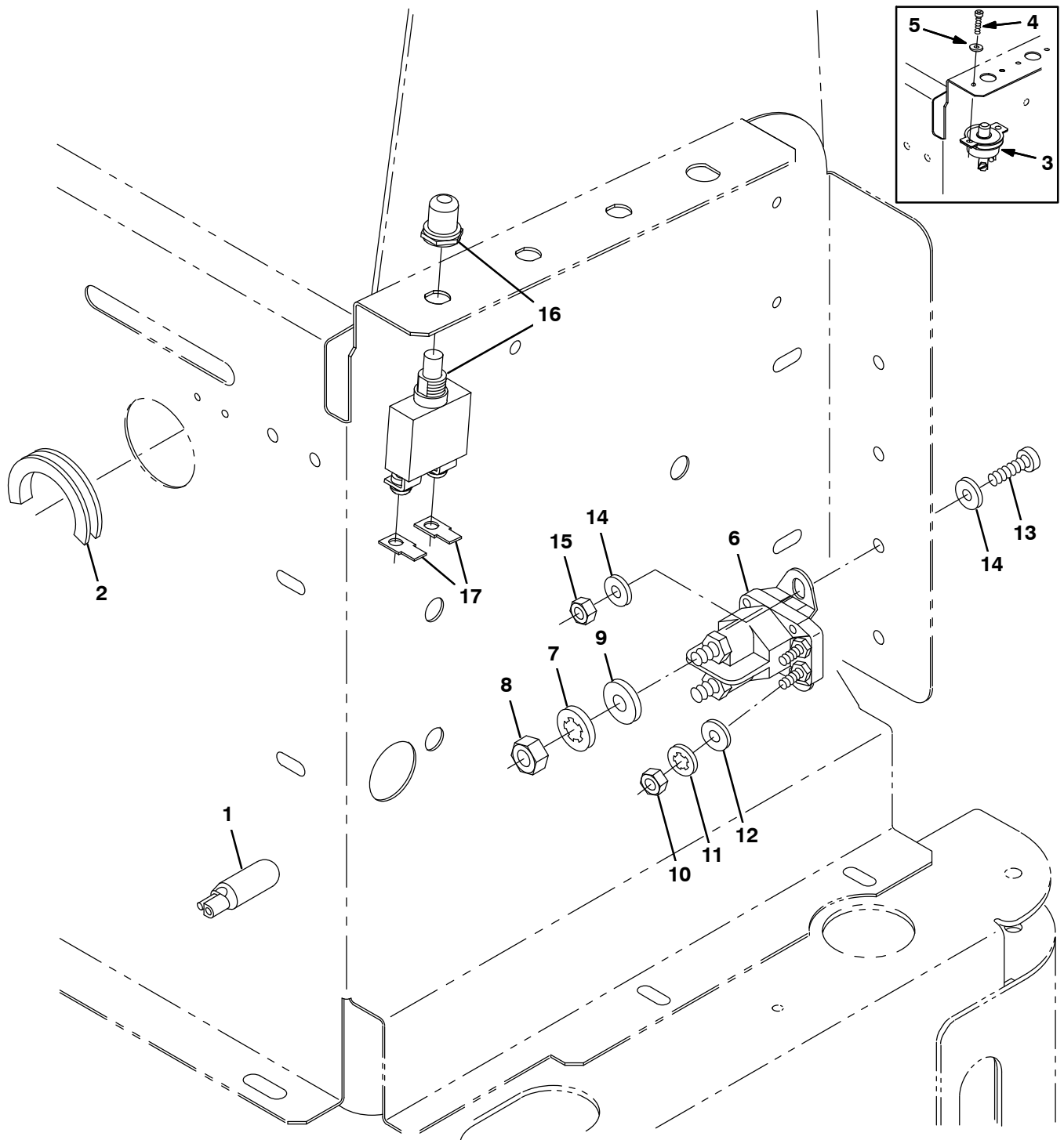
Fig. 6 – Vacuum Wand Electrical Group, Dual Fan — Saugstab-Elektrik-Gruppe, Doppelentlüfter — Système électrique du manche d'aspiration, double extracteur
