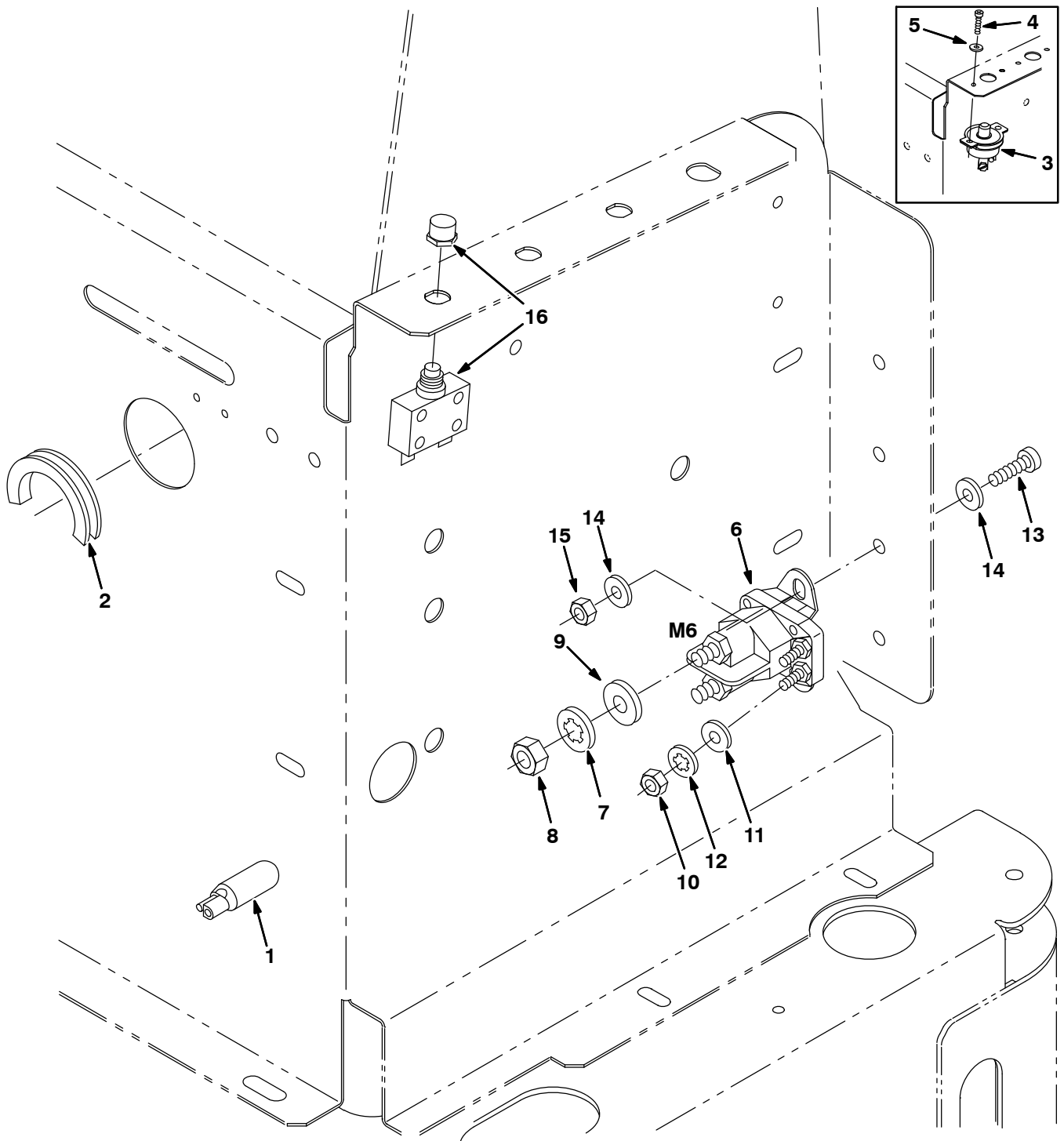
Fig. 4 – Vacuum Wand Electrical Group, Single Fan — Saugstab-Elektrik-Gruppe, Einzelventilator — Système électrique du manche d'aspiration, extracteur simple
