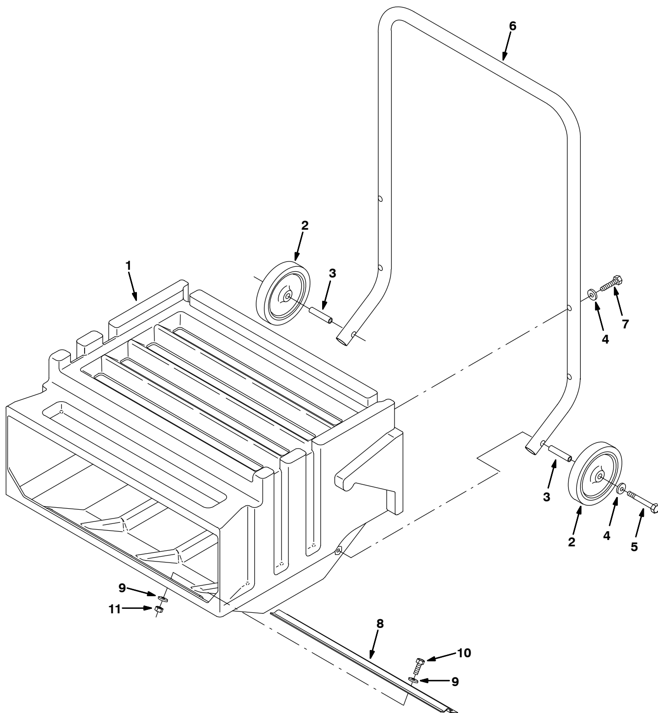
Fig. 26 – Hopper Group — Kehrlichtbehälter-Gruppe — Groupe trémie
