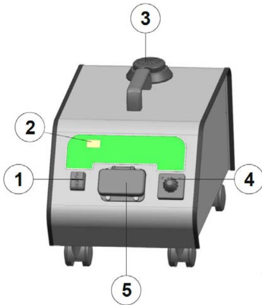
Abb. 3: Gerätebeschreibung SG 36
