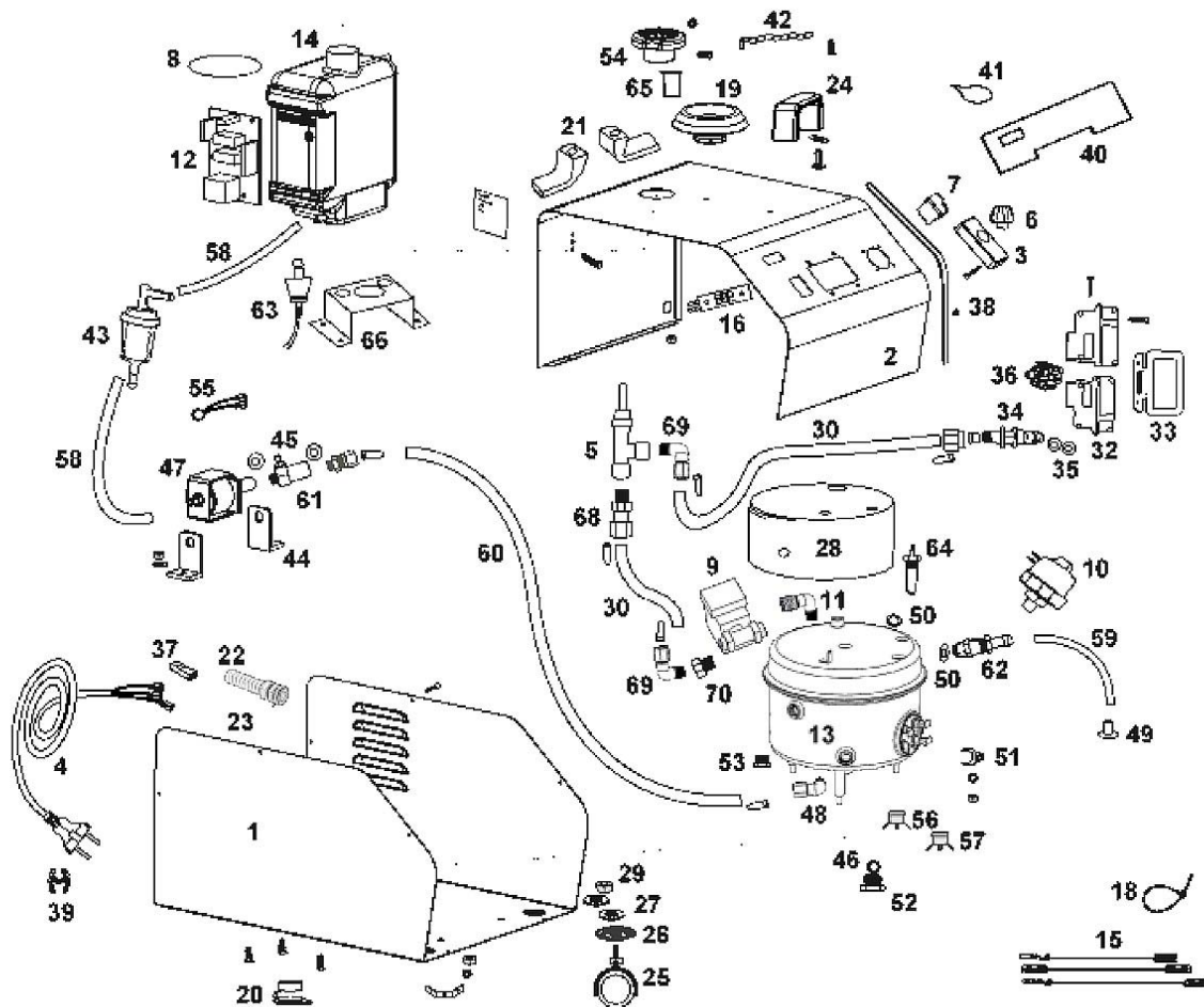
Abb. 17: Ersatzteilzeichnung
