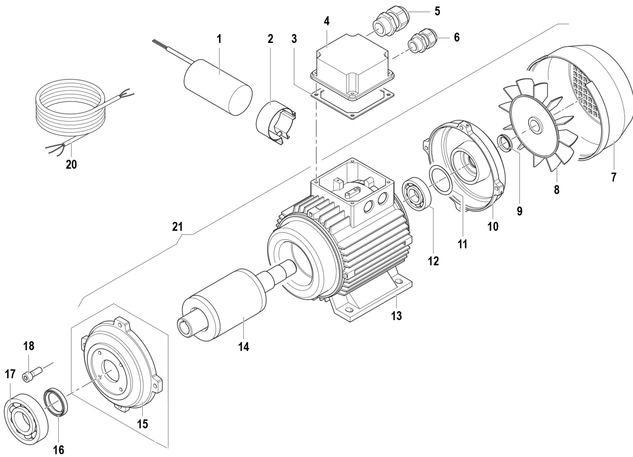
Abb. 2: Ersatzteilzeichnung 2 / Spare parts drawing 2
