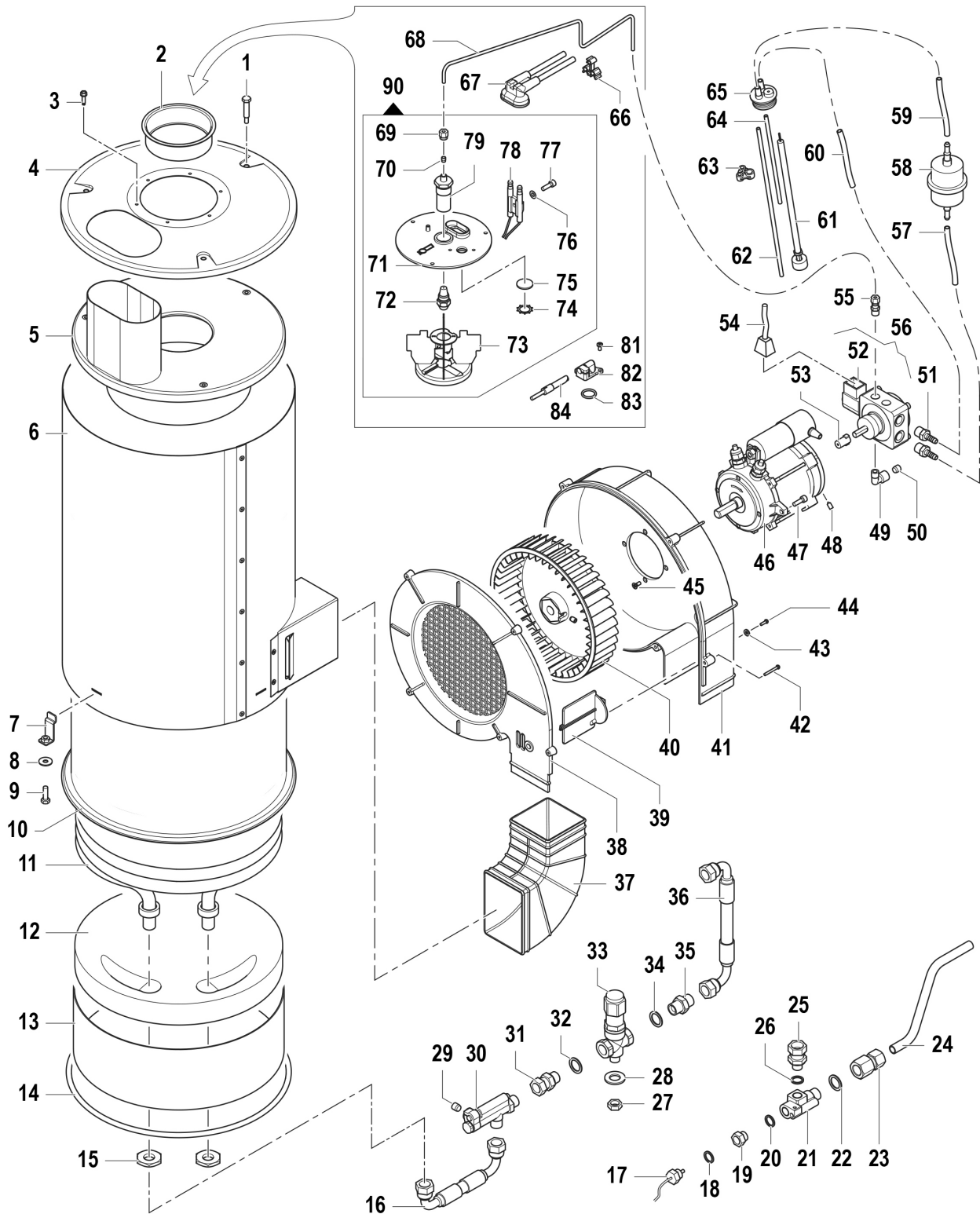
Abb. 8: Ersatzteilzeichnung 8 / Spare parts drawing 8
