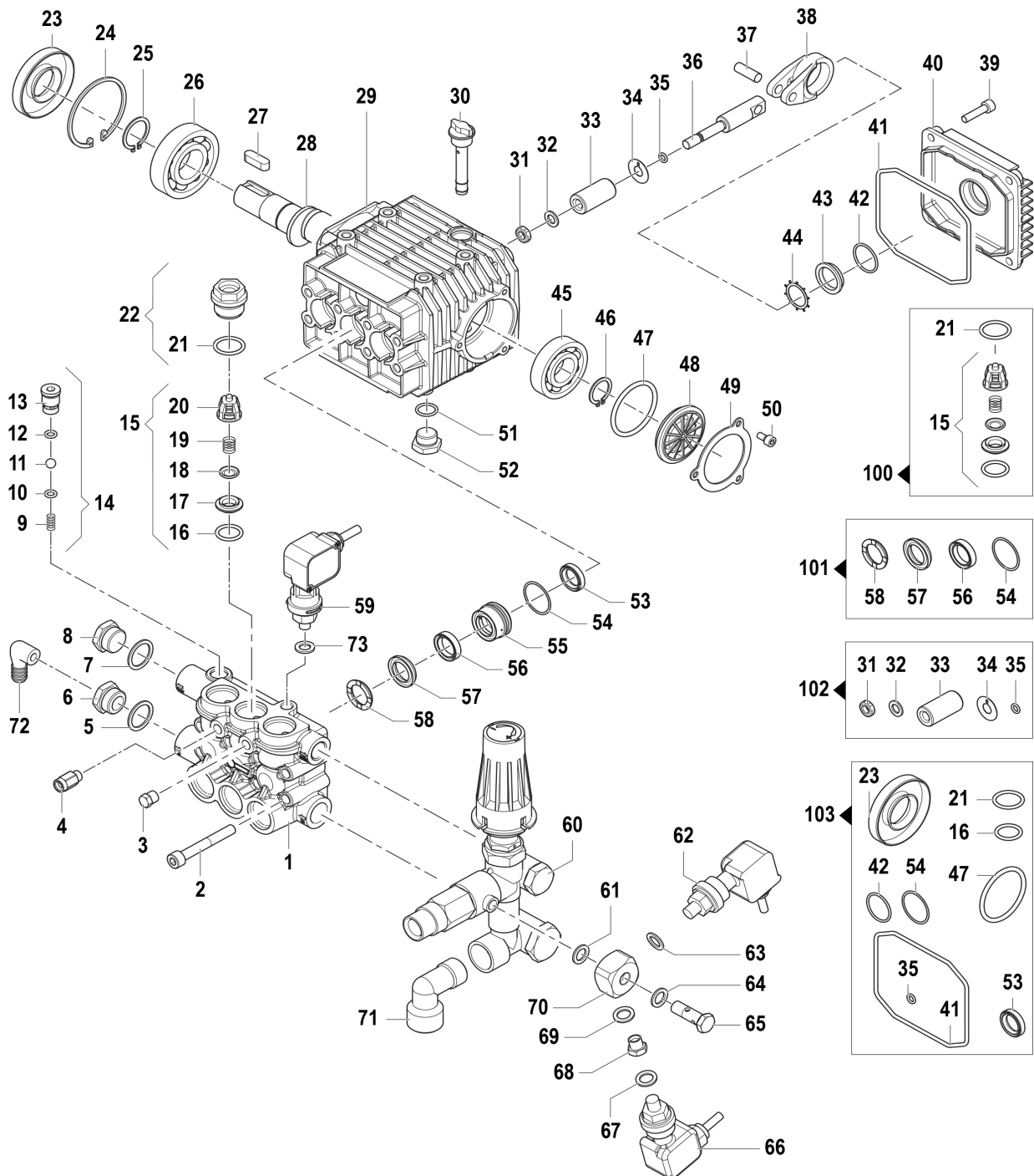
Abb./Fig. 4: Ersatzteilzeichnung 4 / Spare parts drawing 4
