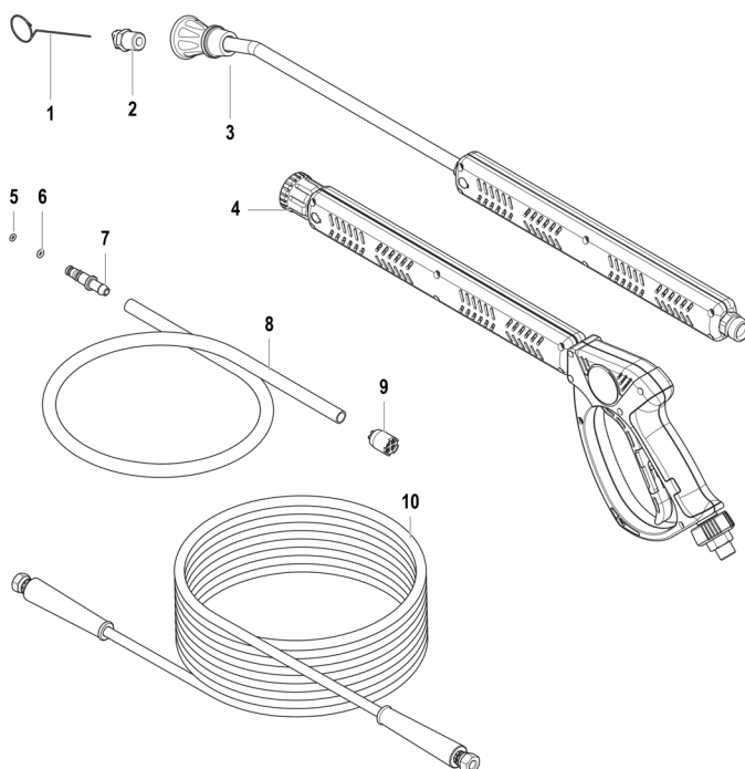
Abb. / Fig. 6: Ersatzteilzeichnung 6 / Spare parts drawing 6
