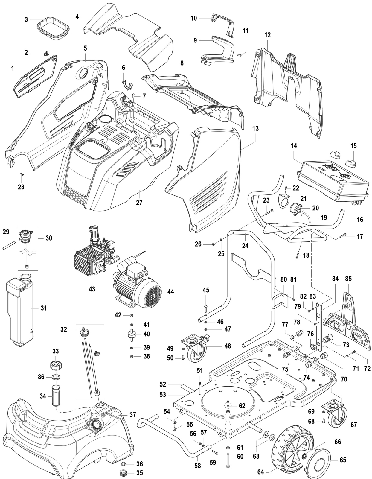
Abb. / Fig. 1: Ersatzteilzeichnung 1 / Spare parts drawing 1
