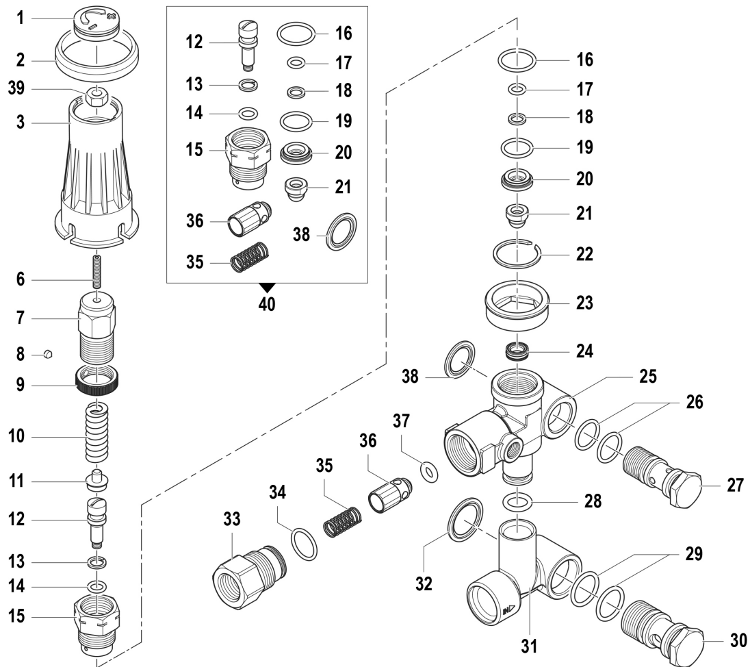
Abb. / Fig. 5: Ersatzteilzeichnung 5 / Spare parts drawing 5
