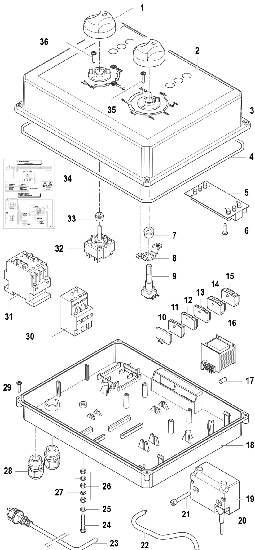
Abb. / Fig. 7: Ersatzteilzeichnung 7 / Spare parts drawing 7
