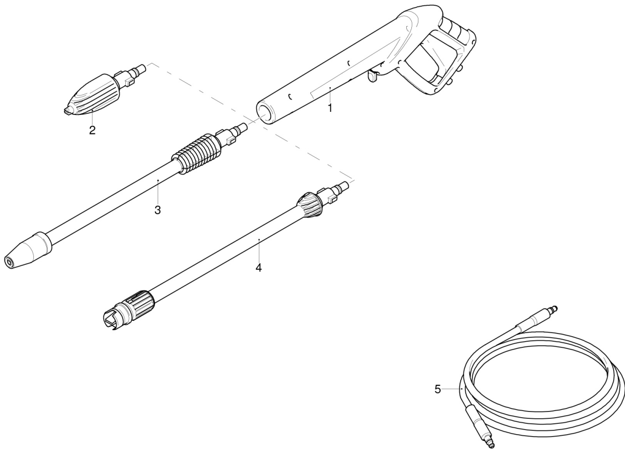
Abb. / Fig. 2: Ersatzteilzeichnung 2 / Spare parts drawing 2
