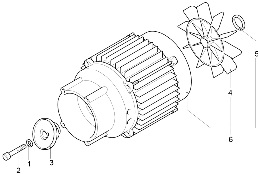
Abb. / Fig. 3: Ersatzteilzeichnung 3 / Spare parts drawing 3
