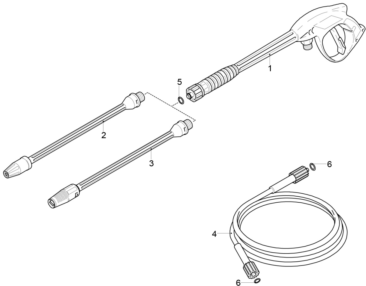
Abb. / Fig. 4: Ersatzteilzeichnung 4 / Spare parts drawing 4
