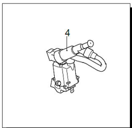
Abb. / Fig. 2: Ersatzteilzeichnung / Spare Parts Drawing 3 oben / above und / and 4 unten / below für / for HDR-K 72-22 BH
