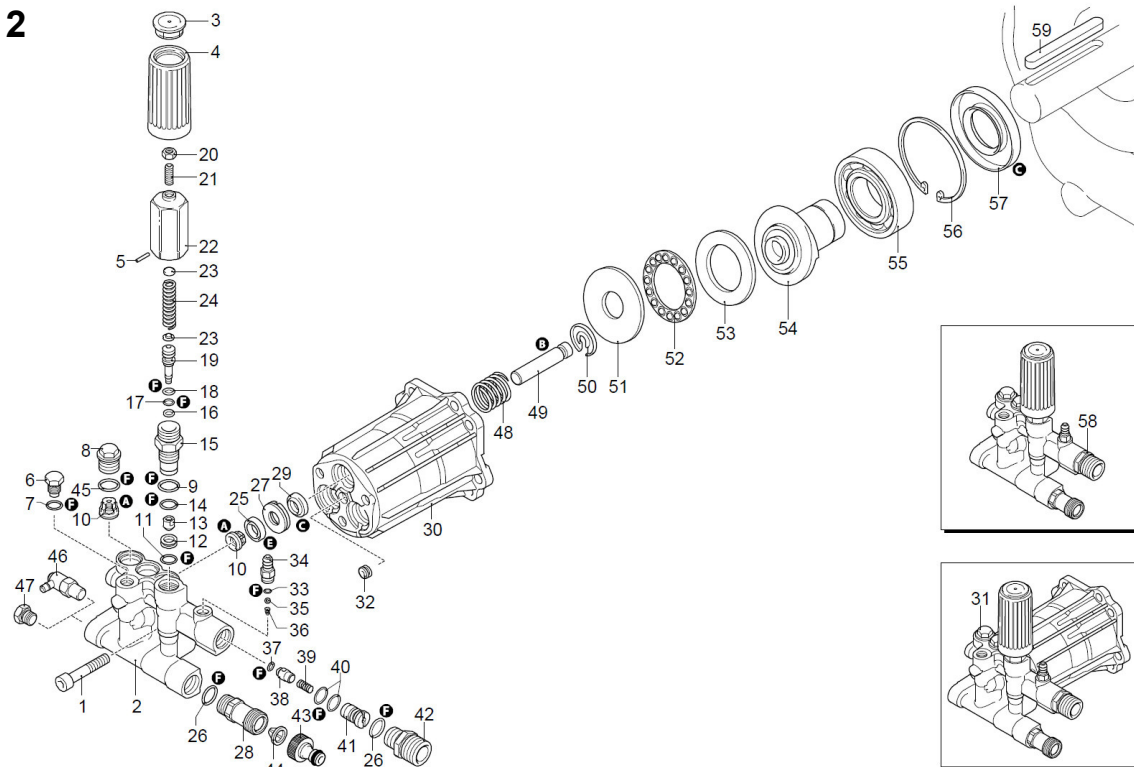
Abb. / Fig. 1: Ersatzteilzeichnung / Spare Parts Drawing 1 oben / above für / for HDR-K 66-20 BL und / and 72-22 BH und / and Ersatzteilzeichnung / Spare Parts Drawing 2 unten / below für / for HDR-K 66-20 BL
