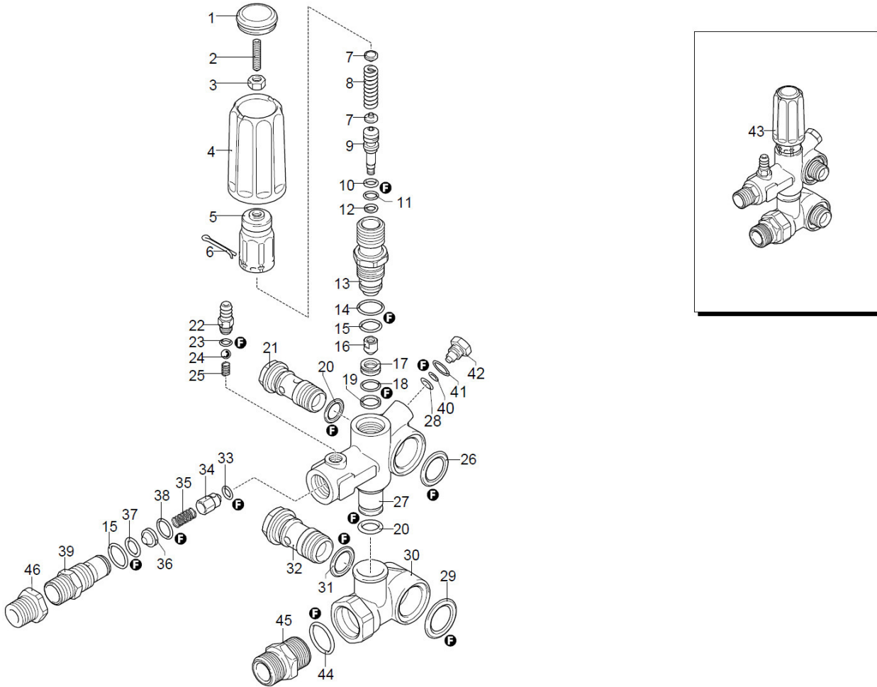
Abb. / Fig. 4: Ersatzteilzeichnung / Spare Parts Drawing 7 für / for HDR-K 96-28 BL
