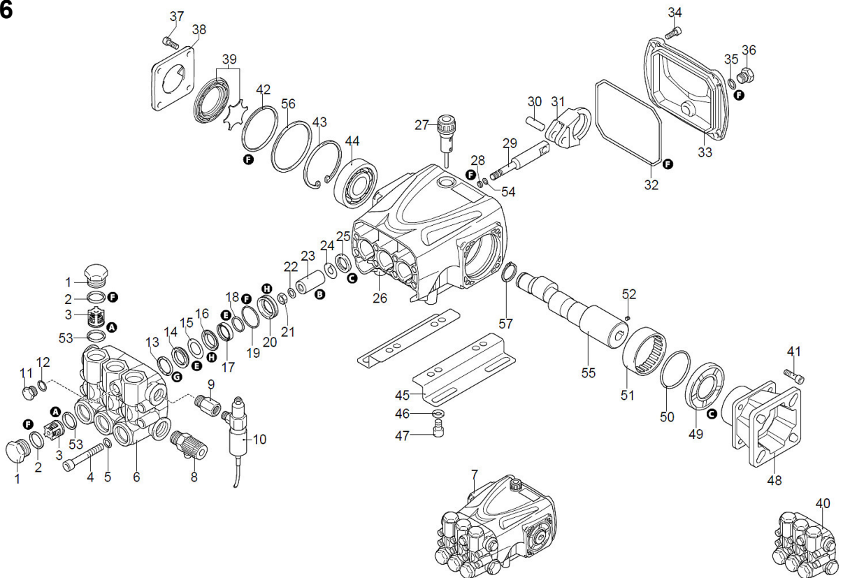
Abb. / Fig. 3: Ersatzteilzeichnung / Spare Parts Drawing 5 oben / above und / and 6 unten / below für / for HDR-K 96-28 BL
