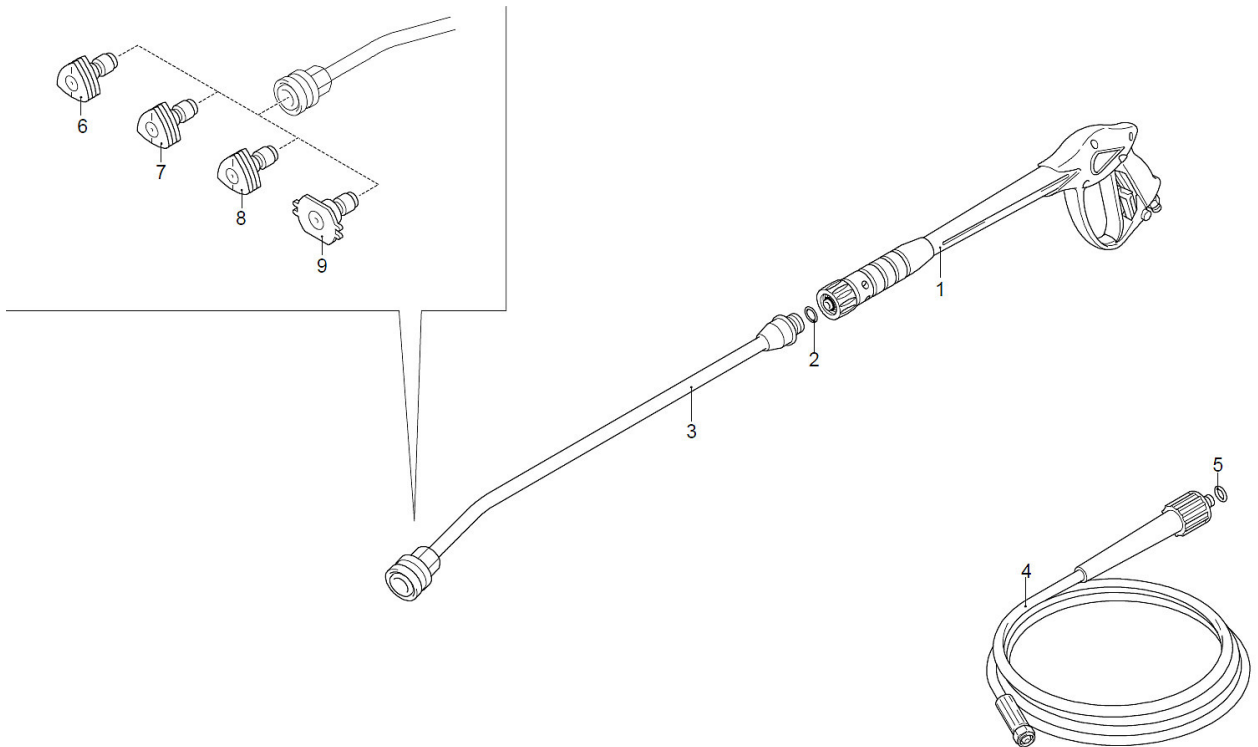
Abb. / Fig. 5: Ersatzteilzeichnung / Spare Parts Drawing 8 für / for HDR-K 66-20 BL / HDR-K 72-22 BH und / and HDR-K 96-28 BL
