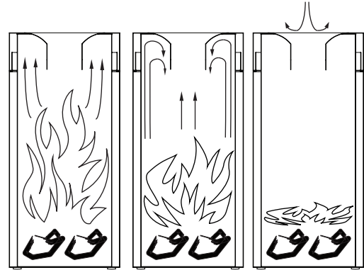
Self-extinguishing functionality / Funktion der Flammverlöschung
