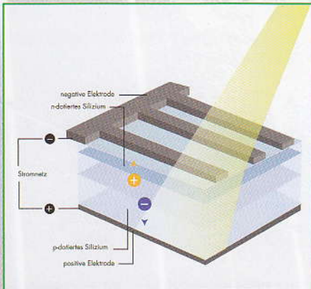
Abb. 1: Funktionsprinzip
