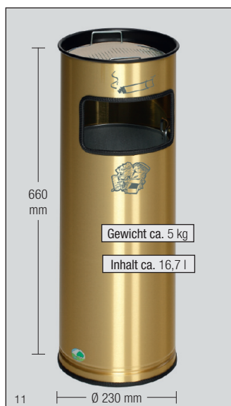
Abb.: „Kombi-Ascher“ H 66 Messing/Stahl-Ausführung Art.-Nr. 1190
