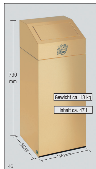
Abb.: „Abfallsammler“ 45-L Messing-Ausführung Art.-Nr. 1198
