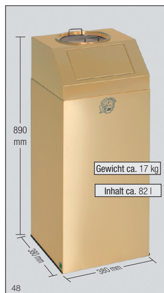
Abb.: „Kombi-Ascher“ 76-L Messing-Ausführung Art.-Nr. 1197
