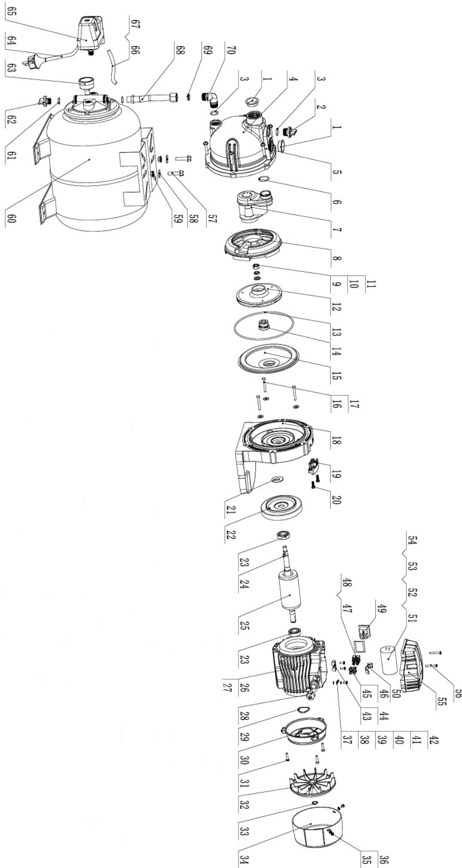
Abb. / Fig. 2: Ersatzteilzeichnung DWS 1105 P / Spare parts drawing DWS 1105 P
