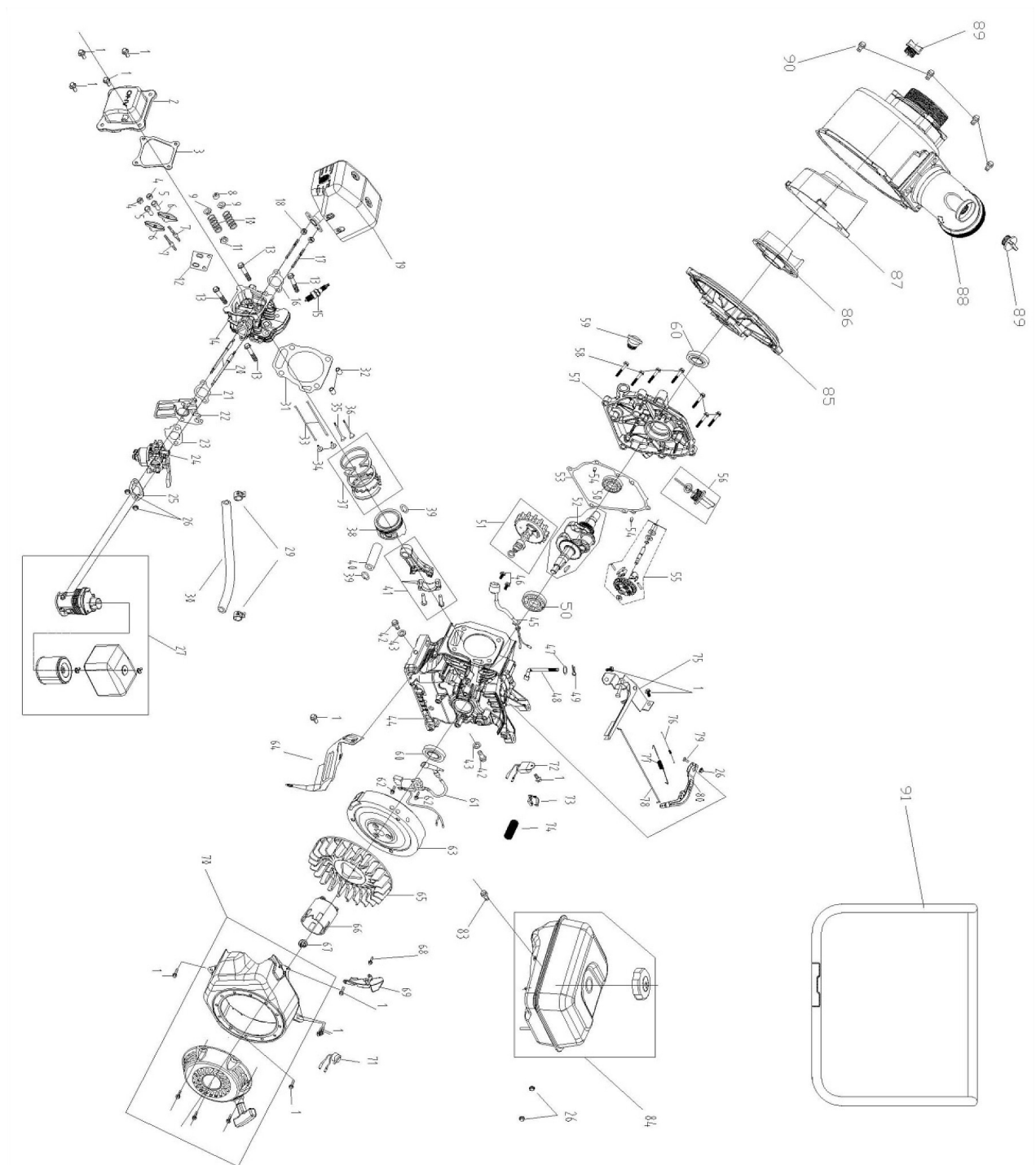
Abb. / Fig. 1: Ersatzteilzeichnung FWP 50 & 80/ Spare parts drawing FWP 50 & 80
